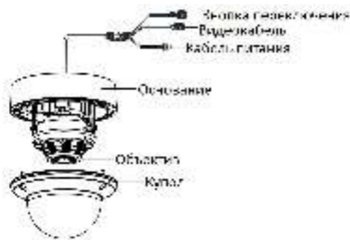
Рисунок 1-2 Камера II типа
