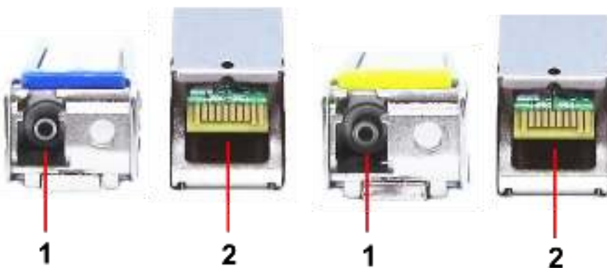
Рис. 4 SFP модули SFP-S1LC19-G-1310-1550, SFP-S1LC19-G-1550-1310, разъемы
