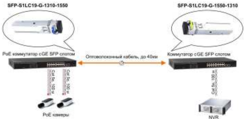
Рис.8 Типовая схема подключения SFP модулей SFP-S1LC19-G-1310-1550, SFP-S1LC19-G-1550-1310
