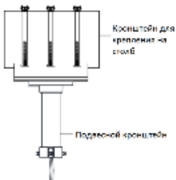
Рисунок 2-6 Установленные кронштейн для крепления на столб и подвесной кронштейн
