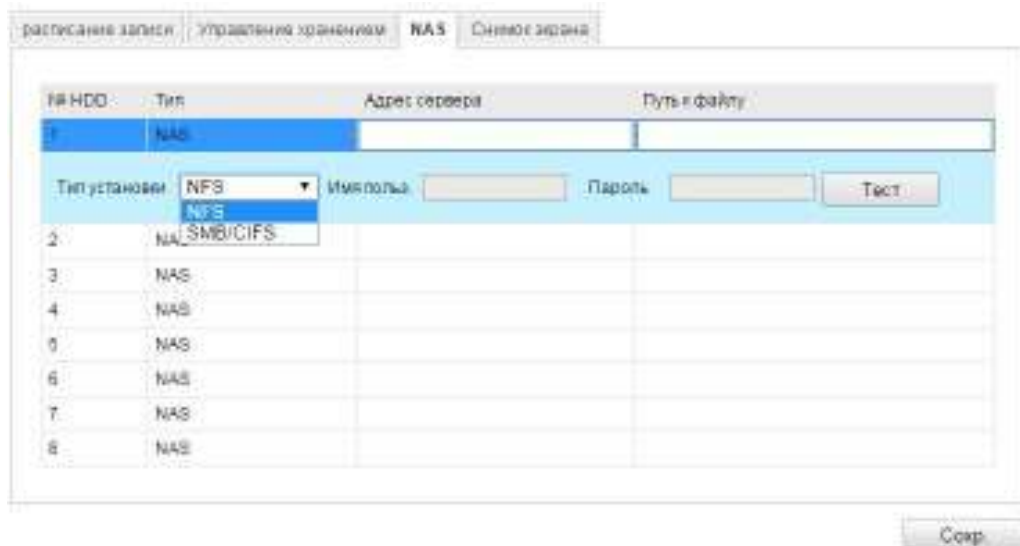
Рисунок 7-1 Добавление сетевого диска
