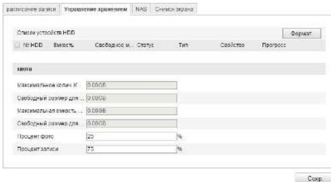
Рисунок 7-2 Инициализация диска
