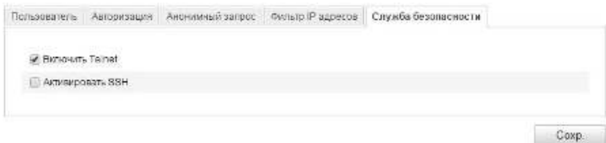
Рисунок 11-8 Служба безопасности
