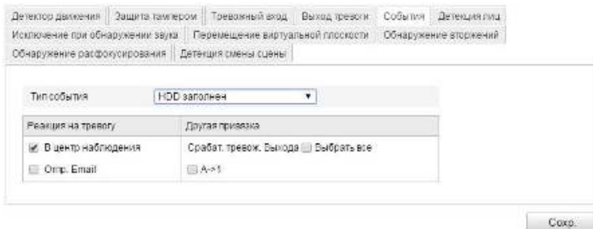
Рисунок 6-42 Настройки событий
