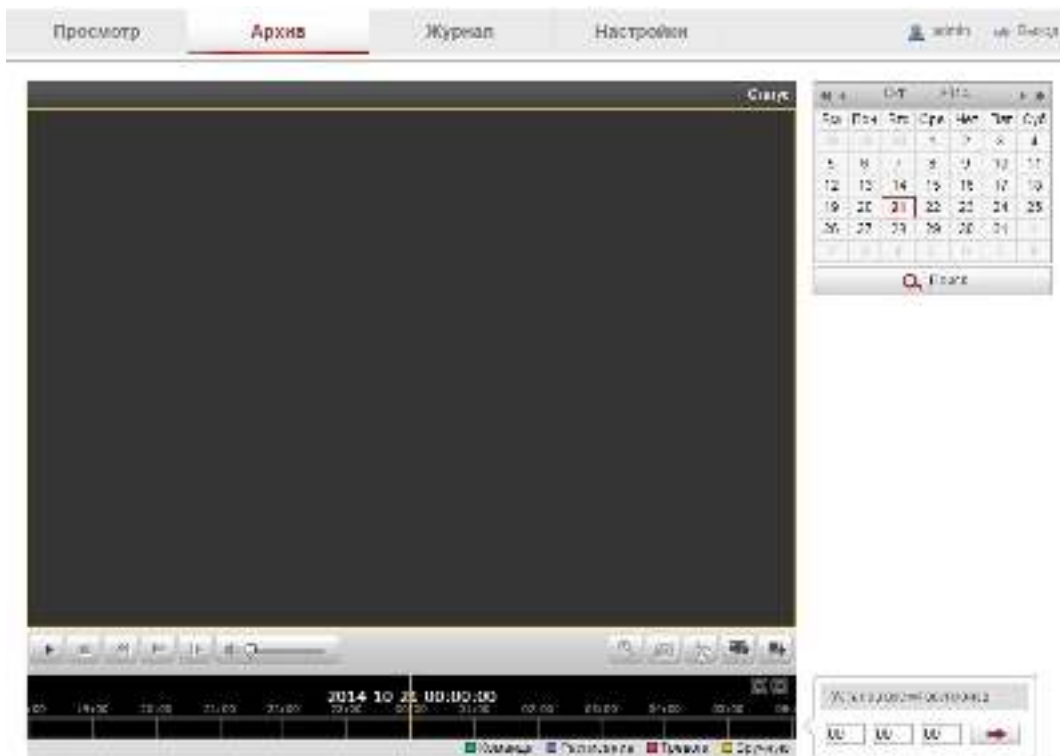
Рисунок 9-1 Интерфейс воспроизведения
