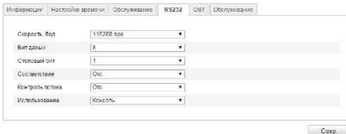
Рисунок 11-12 Настройки RS-232
