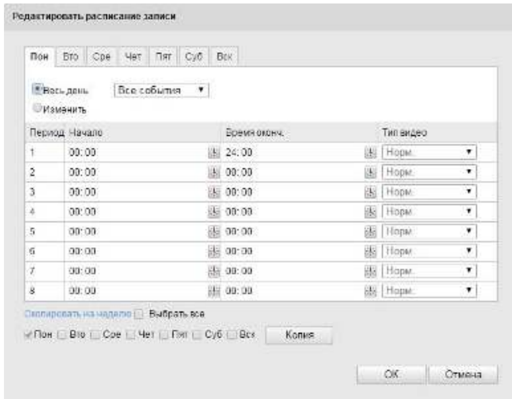
Рисунок 7-4 Расписание записи
