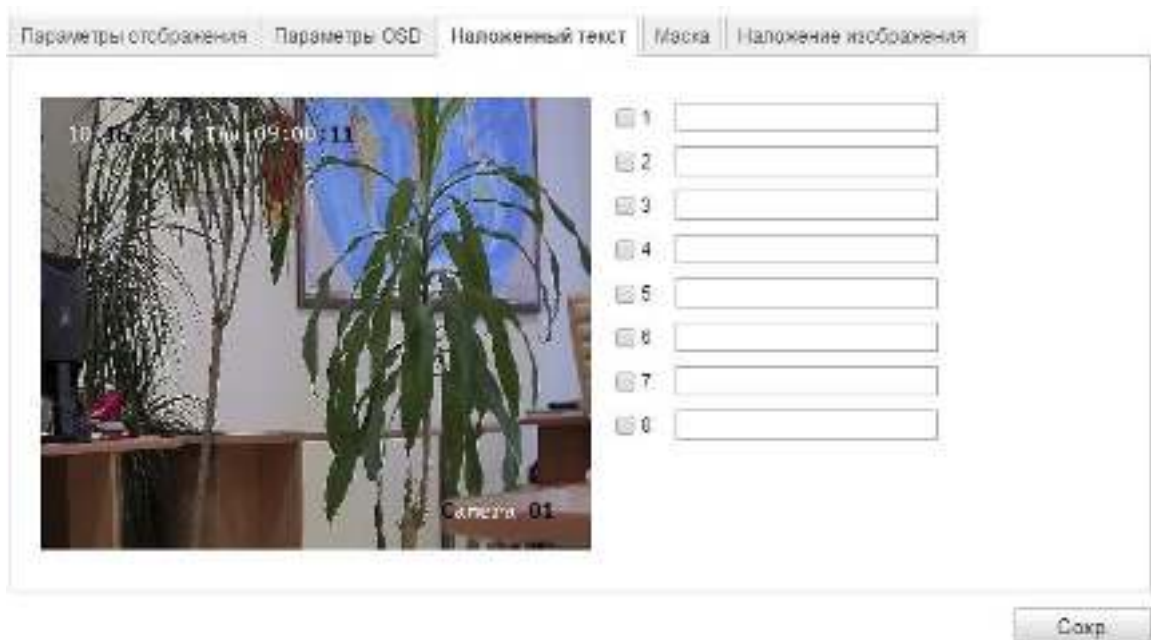
Рисунок 6-30 Наложение текста
