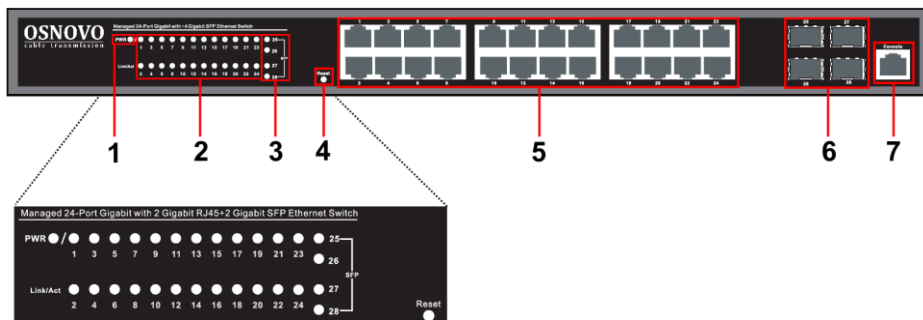
Рис.2 Коммутатор SW-24G4SF-L2, разъемы, кнопки и индикаторы на передней панели
