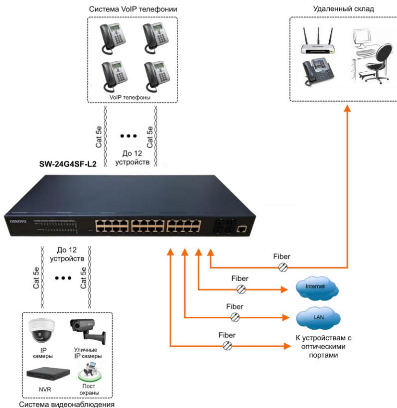
Рис.4 Схема подключения коммутатора SW-24G4SF-L2 на примере сети для небольшого офиса
