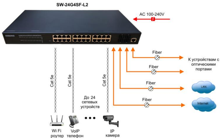
Рис.5 Типовая схема подключения коммутатора SW-24G4SF-L2
