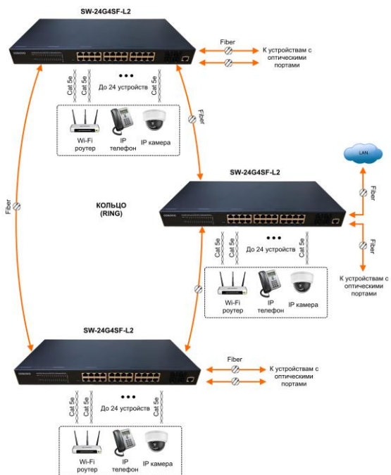
Рис.6 Схема подключения коммутатора SW-24G4SF-L2 при работе в кольцевой топологии
