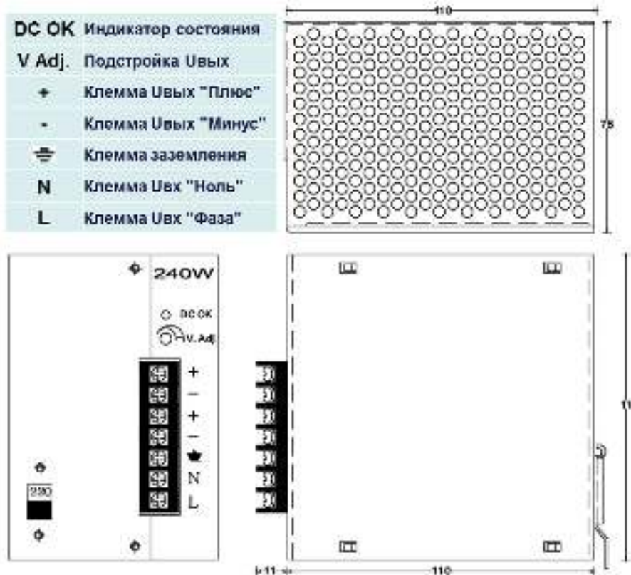
Габаритные размеры AD1360S и обозначения на передней панели
